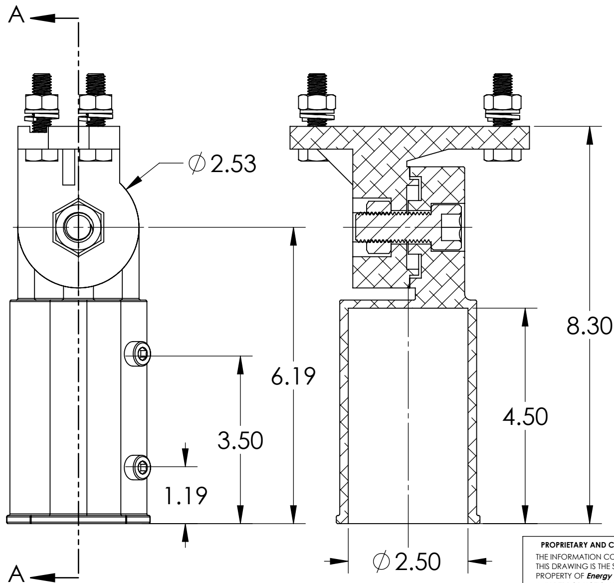
SECTION A-A
